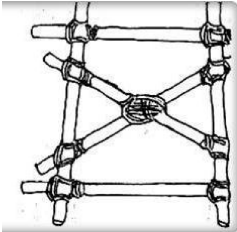
ภาพการผูกแน่นต่อม่อสะพาน
